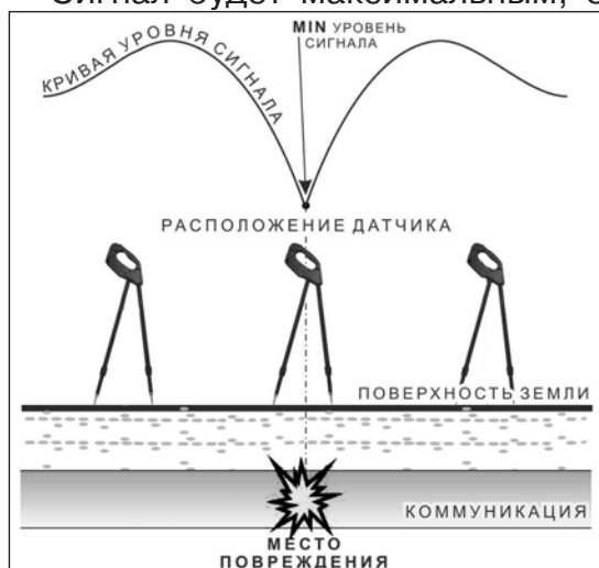
применение датчика контроля изоляции (ДКИ) методом max
