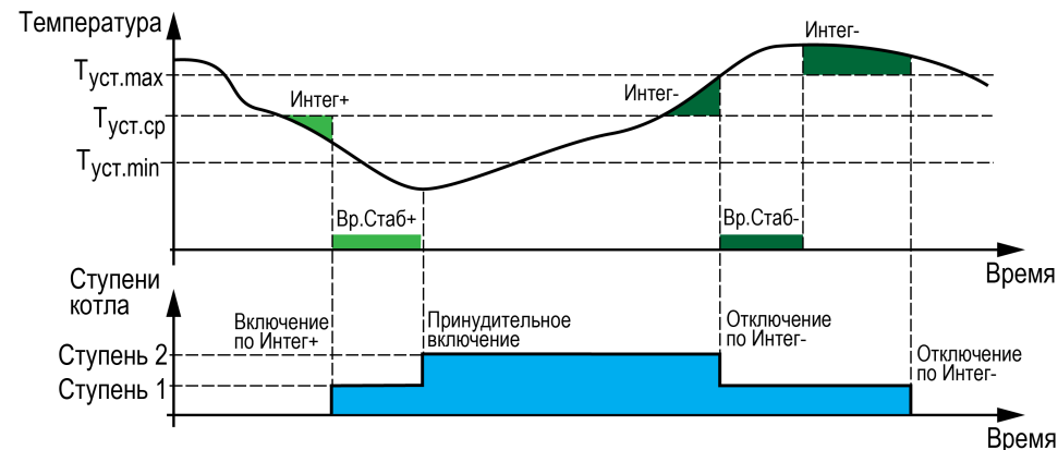
Рисунок 10.2 – Регулирование температуры
