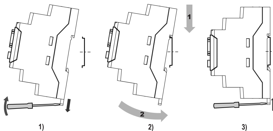
Рисунок 5.2 – Монтаж прибора
