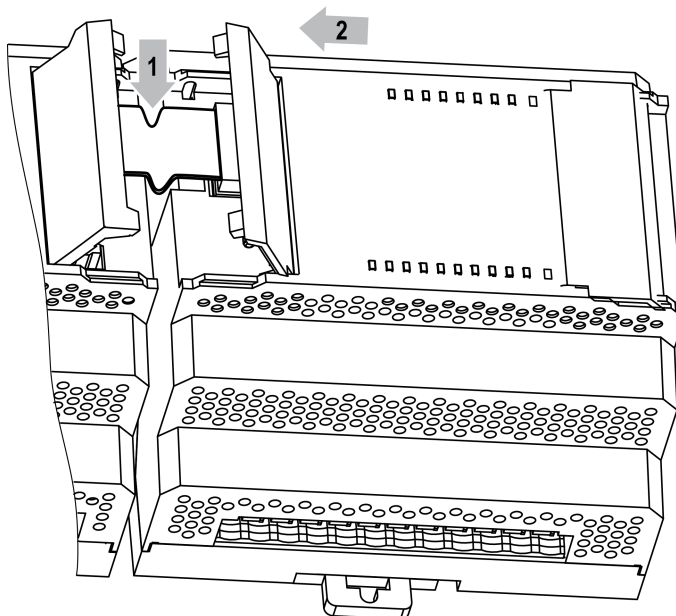
Рисунок 6.16 – Укладка шлейфа в углубление
