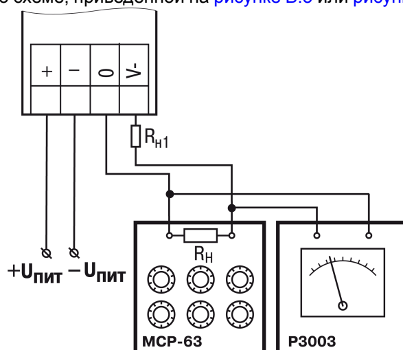
Рисунок В.3 – Схема подключения к ВЭ для юстировки сигналов типа «4...20 мА» ( R_n < 300 \text{ Ом} )
