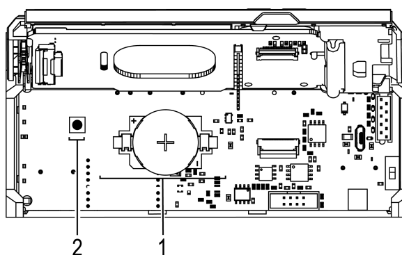
Рисунок 7.3 – Под лицевой панелью
