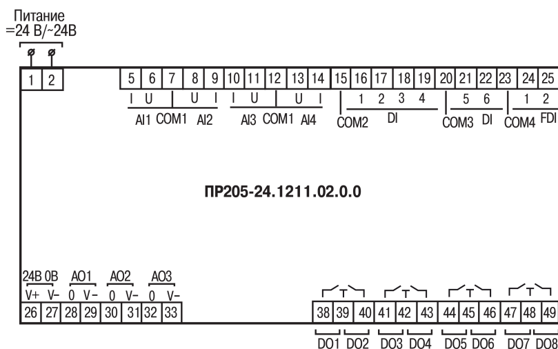
Рисунок А.5 – Расположение контактов для ПР205-24.1211.02.0
