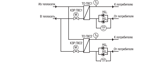
Рисунок 5 – Схема контура «Отопление + ГВС»
