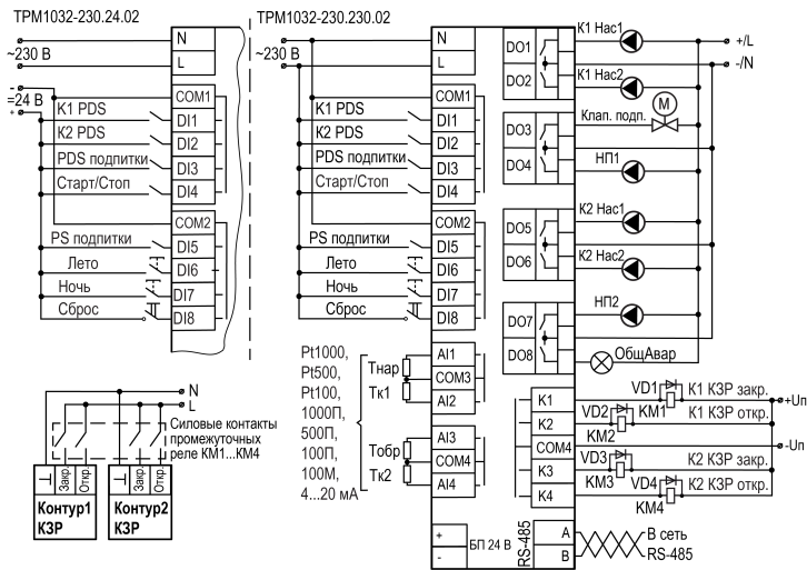
Рисунок 7 – Схема подключения
