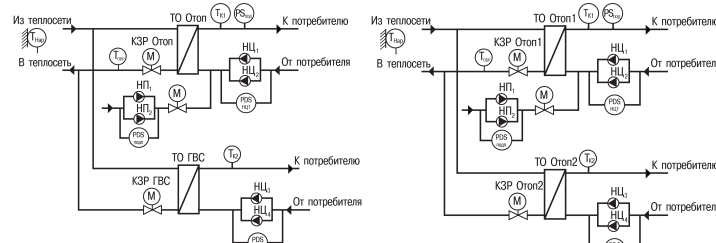
Рисунок 3 – Схема контура «ГВС»
