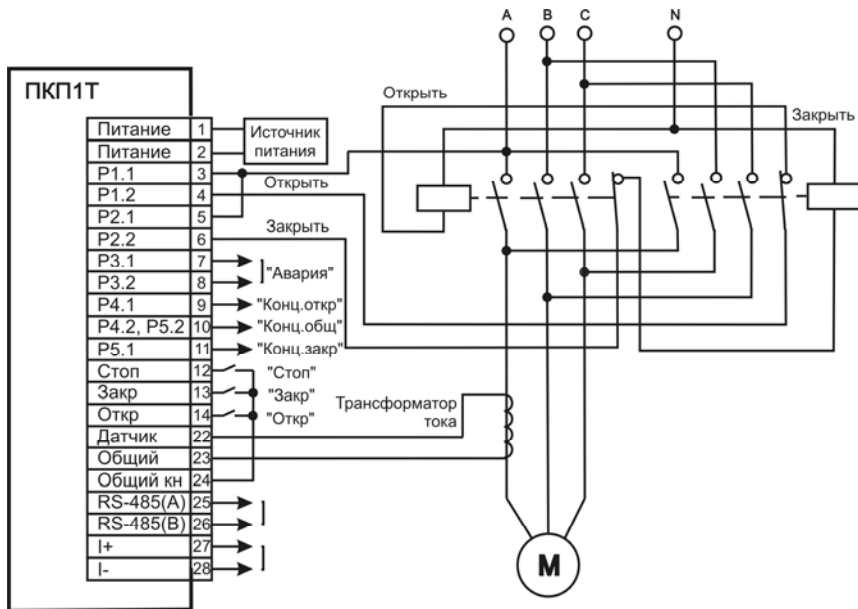
Рисунок Б.2 – Схема подключения прибора
