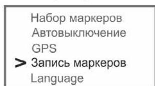
Меню маркероискателя
