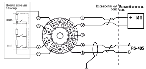
Рисунок 7.3 – Схема подключения с подключением экрана к заземлению
