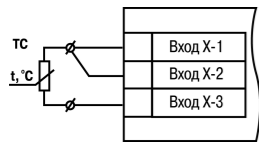
Рисунок 5 – Трехпроводная схема подключения ТС
