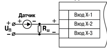
Рисунок 10 – Схема подключения пассивного датчика с токовым выходом 0...5 мА или 0(4)...20 мА R_{ш} = 100,000 \pm 0,025 \text{ Ом}
