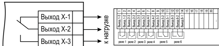
Рисунок 12 – Схема подключения электромагнитных реле прибора ТРМ136-Р
