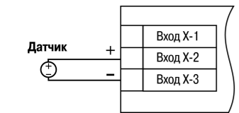
Рисунок 9 – Схема подключения активного датчика с выходом в виде напряжения 0...+50 мВ или 0...1 В
