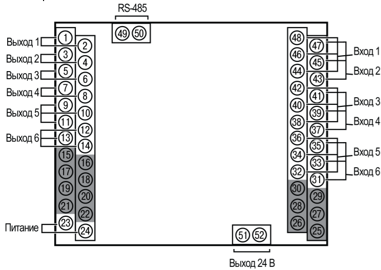
Рисунок 4 – Клеммник ТРМ136-Ц7
