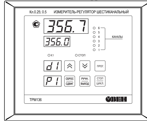
Рисунок 24 – Лицевая панель прибора
