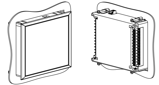
Рисунок 1 – Монтаж прибора щитового крепления
