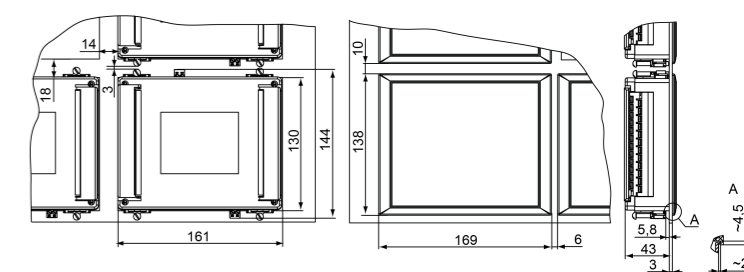
Рисунок 3 – Прибор в корпусе Щ7, установленный в щит толщиной 3 мм
