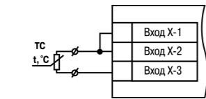
Рисунок 6 – Двухпроводная схема подключения ТС
