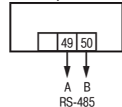
Рисунок 23 – Схема подключения для интерфейса RS-485
