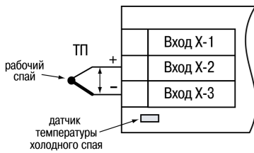
Рисунок 7 – Схема подключения термопары
