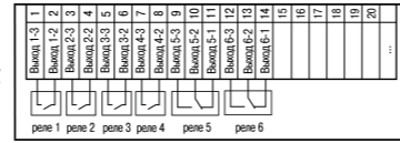
Рисунок 12 – Схема подключения электромагнитных реле прибора ТРМ136-Р
