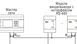
Рисунок 13 – Типовая схема подключения в режиме Master
