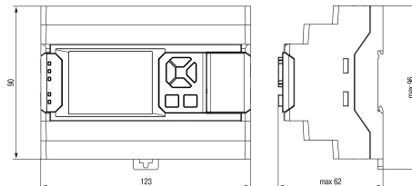
Рисунок 1 – Габаритные размеры прибора
