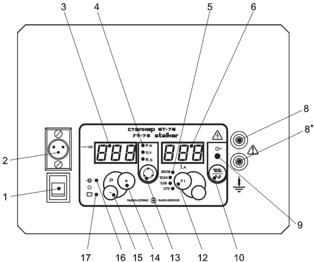
Рисунок 1.4.2 а - Передняя панель генератора ГТ-75
