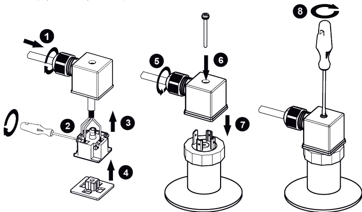
Рисунок 4 – Монтаж проводов
