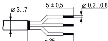
Рисунок 3 – Подготовка кабеля
