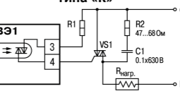
Рисунок 12 – Подключение к ВЭ нагрузки типа «С»
