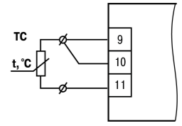
Рисунок 7 – Подключение ТС по трехпроводной схеме
