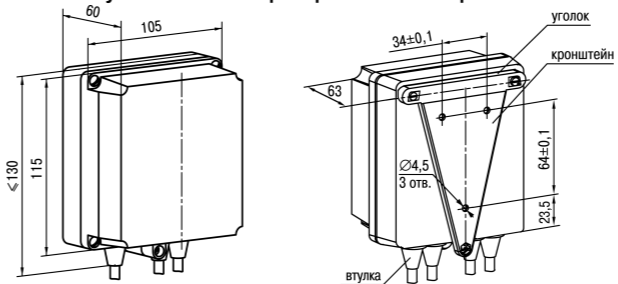
Рисунок 2 – Габаритные размеры корпуса Н
