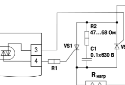
Рисунок 14 – Управление двумя тиристорами, подключенными встречно-параллельно
