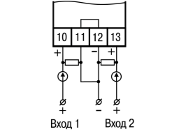
Рисунок 9 – Подключение активных датчиков
