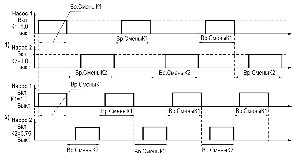
Рисунок 8.3 – Работа насосов при: 1) одинаковых хода, 2) при меньшем втором коэффициенте
