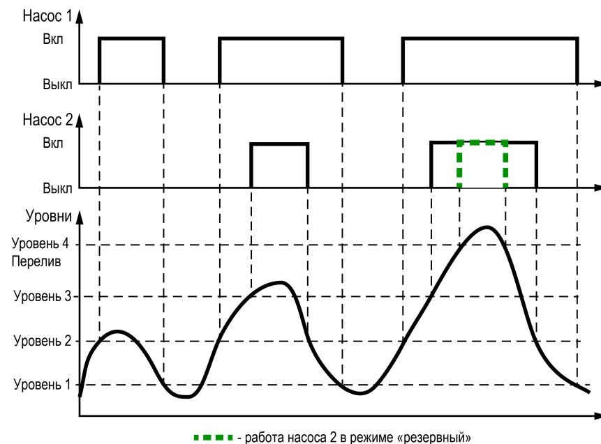
Рисунок 8.1 – Регулирование уровня
