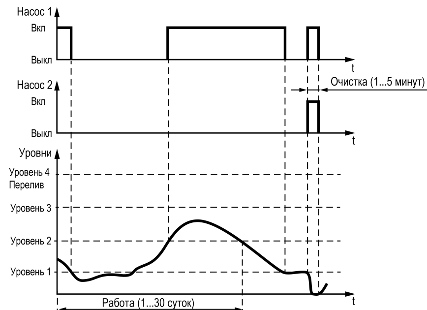
Рисунок 8.4 – Очистка от стоков
