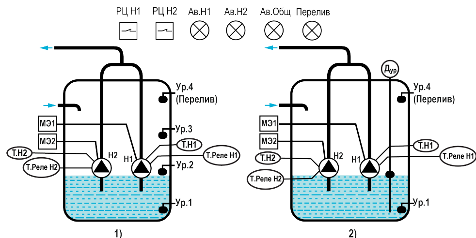
Рисунок 1.1 – Схема объекта управления: 1) с дискретными датчиками уровня, 2) с дискретными и аналоговым датчиками уровня
