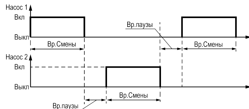
Рисунок 8.2 – Чередование насосов
