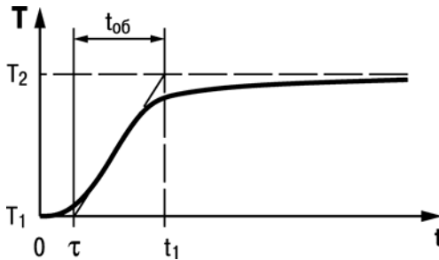
Рисунок Г.2 – График переходной функции
