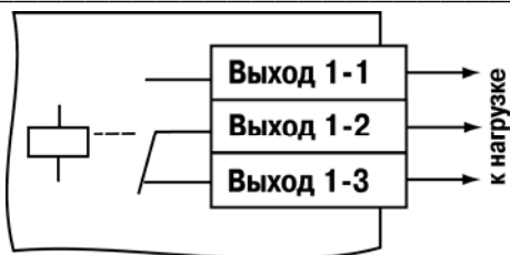
Рисунок Б.8 – Схема подключения нагрузки к ВУ типа P (для первого ВУ)
