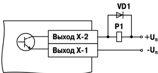
Рисунок Б.9 – Схема подключения нагрузки к ВУ типа K
