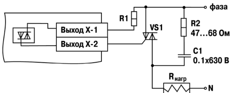
Рисунок Б.10 – Схема подключения нагрузки к ВУ типа C
