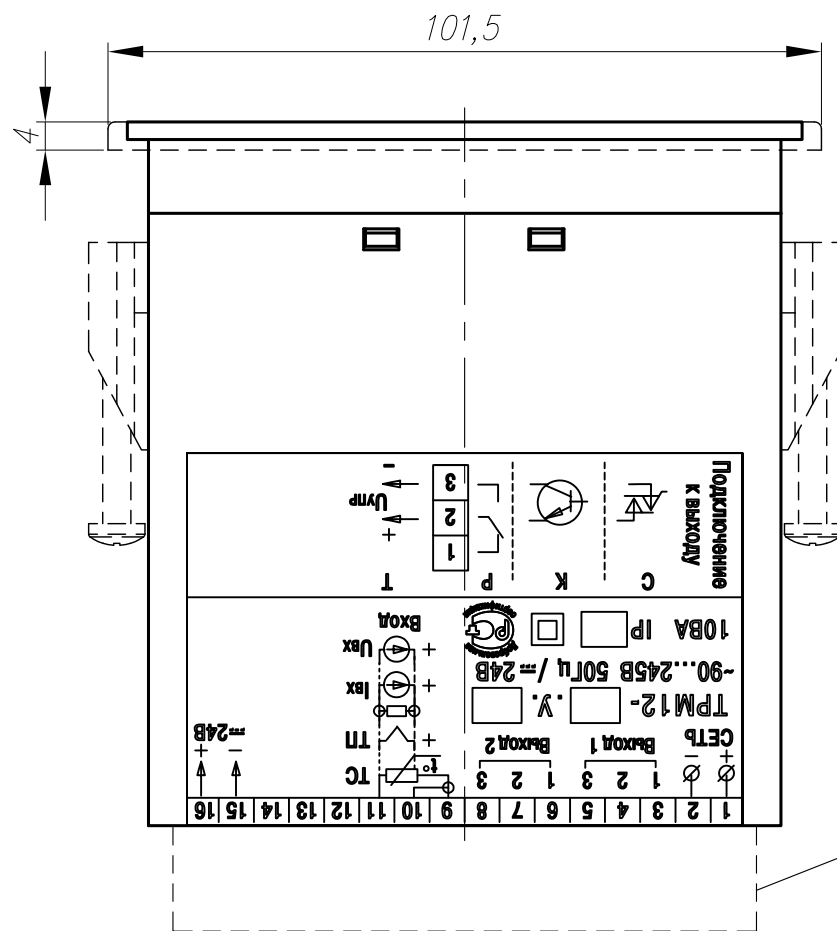
Вид снизу
