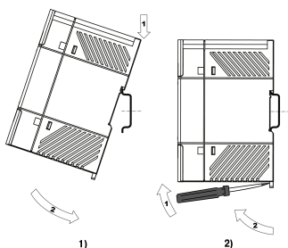
Рисунок 2 - Монтаж (1) и демонтаж (2) прибора
