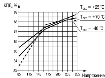
Рисунок 7 - График зависимости КПД от напряжения питания и температуры окружающей среды
