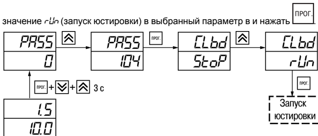
Рисунок 8.2 – Запуск юстировки
