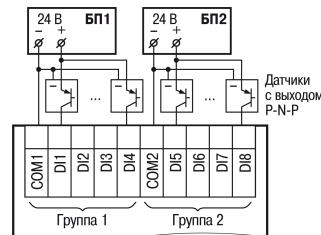
Рисунок 7 – Схема подключения к дискретным входам, работающим в дискретном режиме трехпроводных дискретных датчиков, имеющих выходной транзистор п-р-п-типа с открытым коллектором для сигналов 24 В
