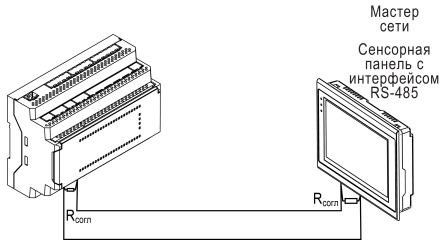
Рисунок 12 – Типовая схема подключения в режиме Slave
