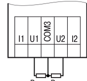
Рисунок 4 – Подключение резистивных датчиков
