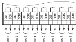
Рисунок 9 – Схема подключения нагрузок к ВЭ типа «Р»
