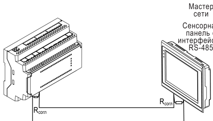
Рисунок 12 – Типовая схема подключения в режиме Slave
