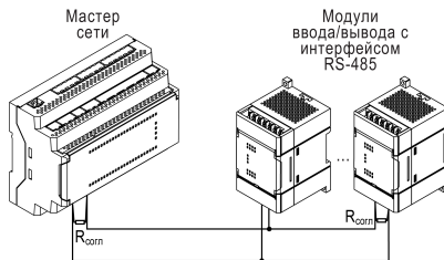
Рисунок 13 – Типовая схема подключения в режиме Master
