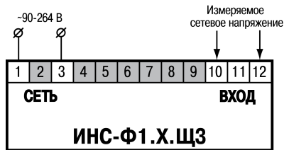
Рисунок 6 – Назначение клеммника прибора модификации ШЗ
