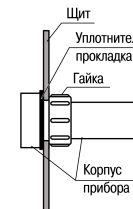
Рисунок 3 – Монтаж прибора щитового крепления
