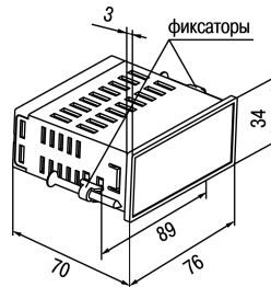
Рисунок 4.2 – Габаритные размеры корпуса ЦЗ
