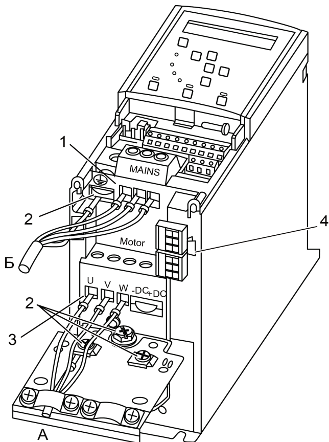
Рисунок 4.3 – Подключение электродвигателя (кабель А, клеммы «Motor») и сетевых проводов (кабель Б, клеммы «Mains»). Цифрами обозначены: 1 – фаза; 2 – заземление; 3 – электродвигатель; 4 – реле
