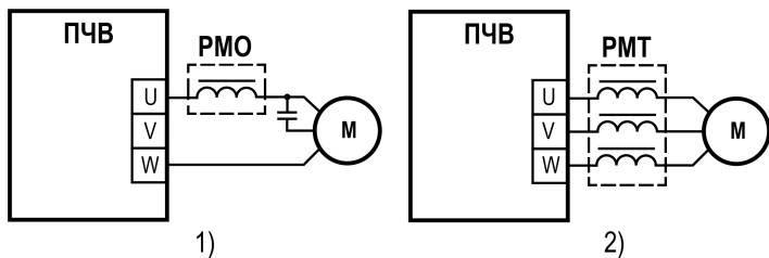
1) серии РМО в выходных цепях ПЧВ для питания однофазных электродвигателей; 2) серии РМТ в выходных цепях ПЧВ для питания
