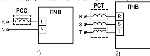
1) серии РС0 во входных цепях питания ПЧВ с однофазным входом; 2) серии РСТ во входных цепях питания ПЧВ с трехфазным входом
