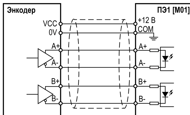
Рисунок 8.10 – Схема подключения энкодера с дифференциальным выходом
