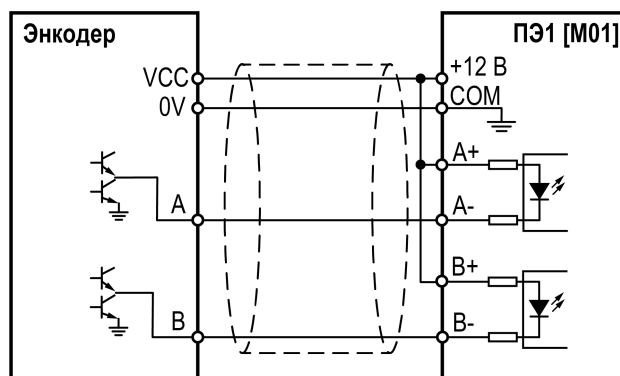
Рисунок 8.12 – Схема подключения энкодера с выходом типа "открытый коллектор"
