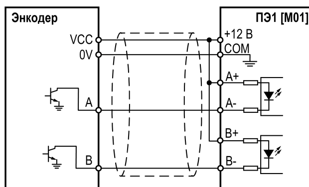
Рисунок 8.11 – Схема подключения энкодера с выходом типа "открытый коллектор"
