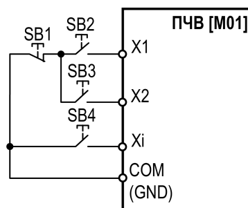
Рисунок 8.6 – Трехпроводная схема управления 1 (F05.20 = 2)
