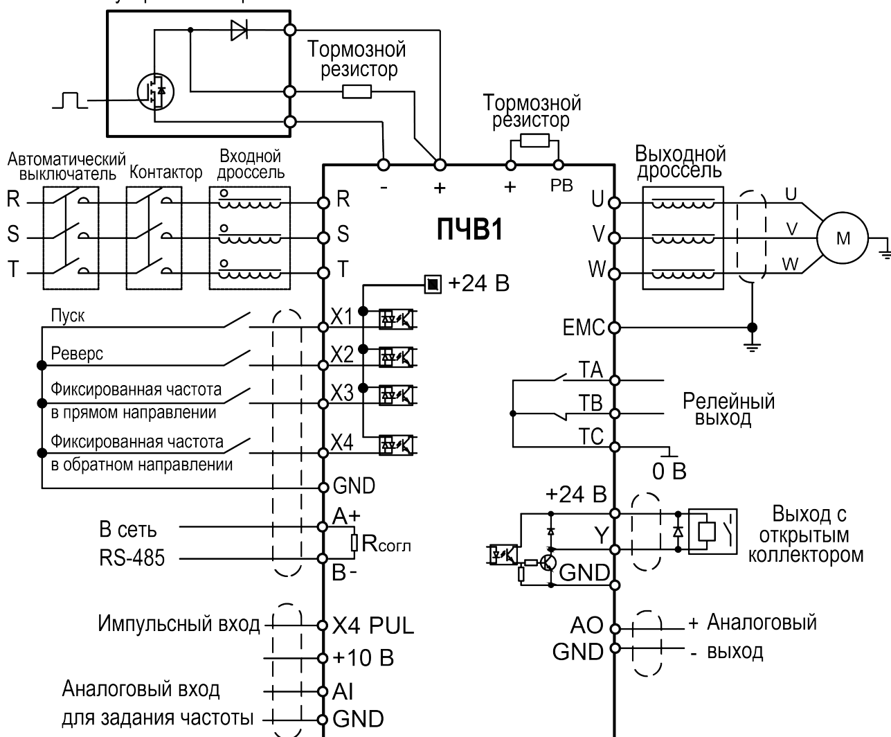
Рисунок 6.6 – Общая схема подключения
