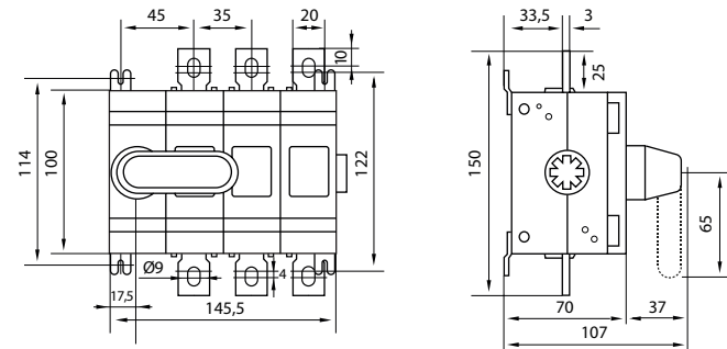
Рис. 1 - Выключатель-разъединитель ВНК-35-1
