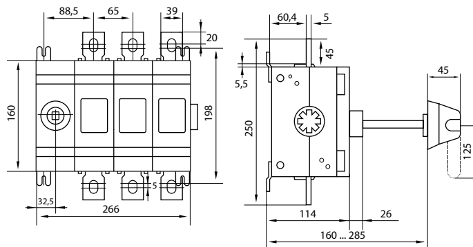
Рис. 6 - Выключатель-разъединитель ВНК-37-2
