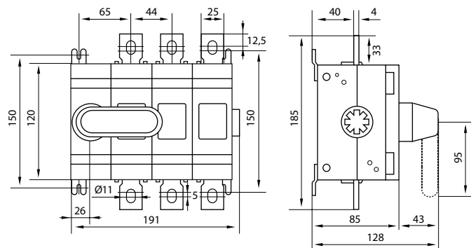
Рис. 3 - Выключатель-разъединитель ВНК-37-1
