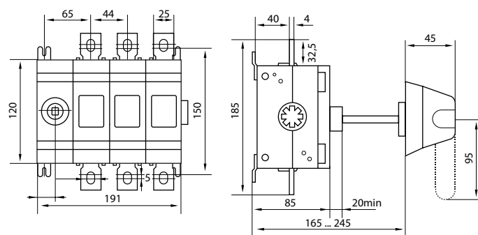
Рис. 4 - Выключатель-разъединитель ВНК-37-2
