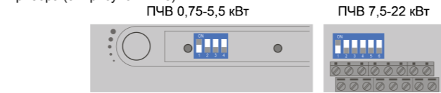
Рисунок 4 – Вид на блок DIP-переключателей
