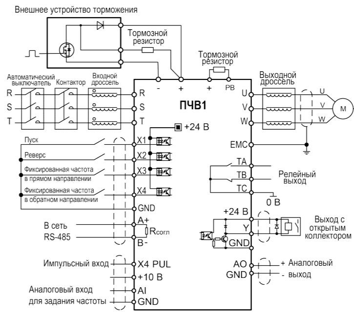
Рисунок 7 – Общая схема подключения
