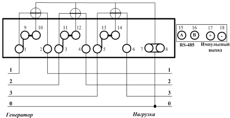
Схема непосредственного включения счётчика
