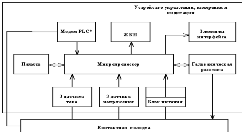
Рис. 1 Обобщённая структурная схема счётчика
