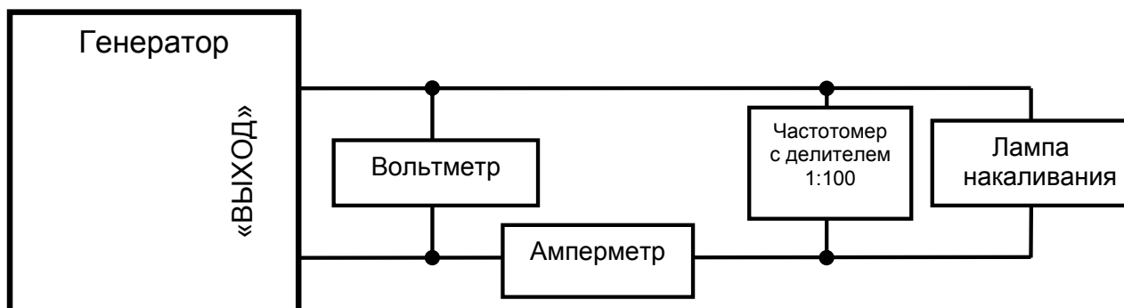
Рисунок 7.5.3 – Схема рабочего места для проверки параметров генератора
