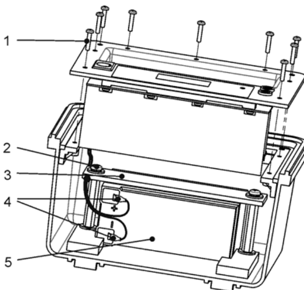
Рисунок 3.3 - Внутренняя конструкция генератора ГТ-15
