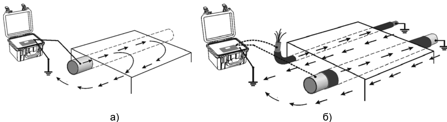
Рисунок 2.3.1 –Подключение генератора к коммуникациям:
