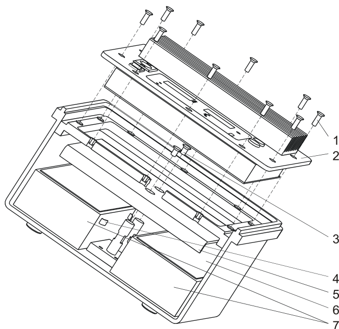
Рисунок 3.2 - Внутренняя конструкция генератора ГТ-75
