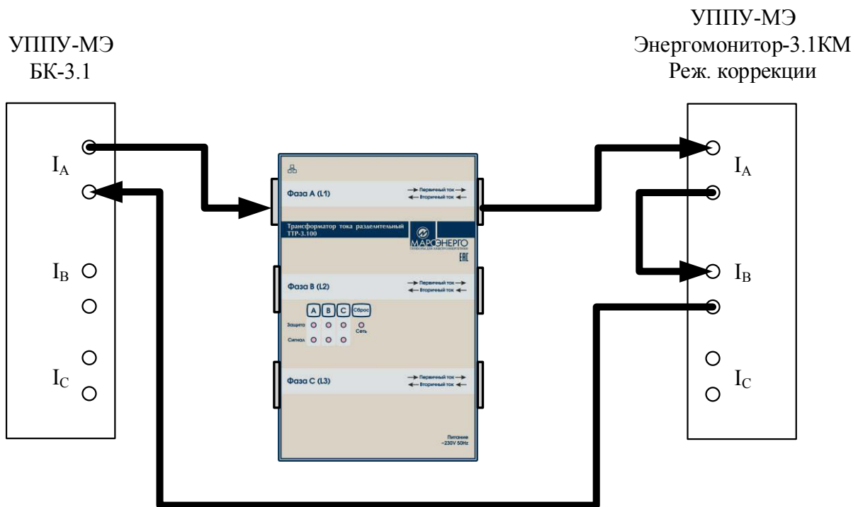
Рисунок 4.7.6а – Схема подключения разделительного ТТ в режиме коррекции измерительных каналов прибора
