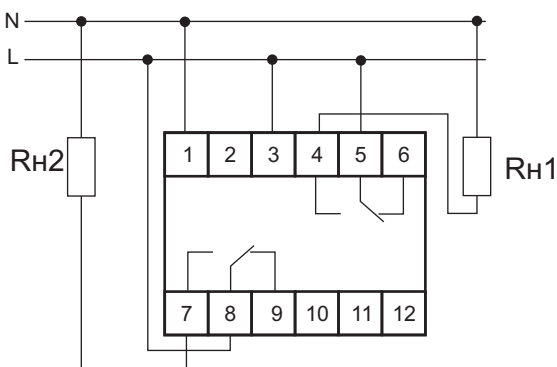
Rn1 и Rn2 - подключаемая нагрузка
