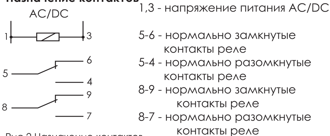
Рис.2 Назначение контактов.
