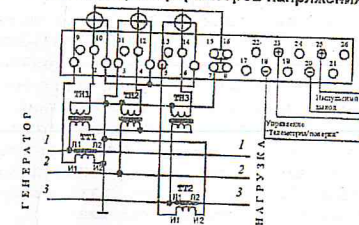
Схема подключения счётчика к трёхфазной 3-проводной сети с помощью трёх трансформаторов напряжения и двух трансформаторов тока.
