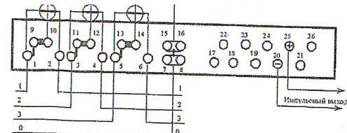
Схема непосредственного подключения счётчика.
