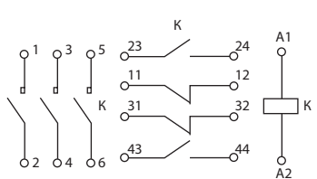
Рис. 1 - Пускатели серии ПМА 3100, 3110
