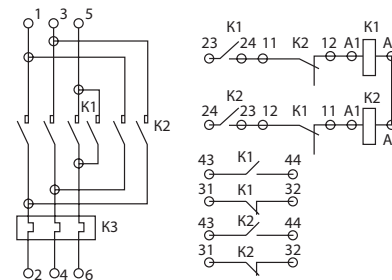
Рис. 3 - Пускатели серии ПМА 3300
