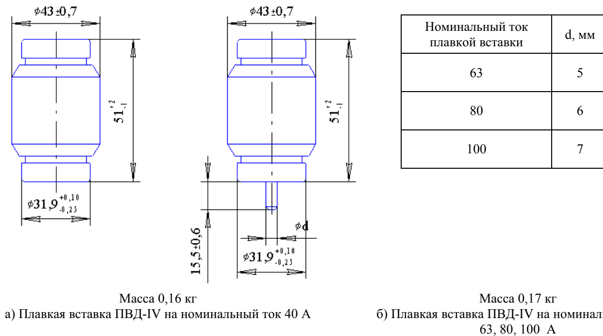
Рис. 15.2 - Плавкая вставка ПВД-IV
