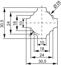
ТШП-0,66 габарит 30(Т)
