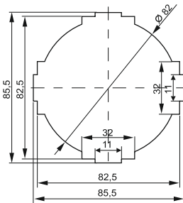
Рисунок 3 – Размеры отверстий под шины и кабели.
