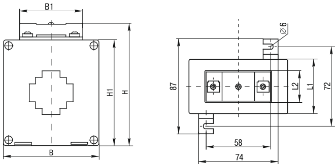
Рисунок 2 – Габаритные и установочные размеры трансформаторов ТШП-0,66.
