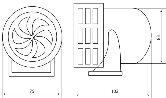
Рис. 2 - Сирена серии CC-1K
