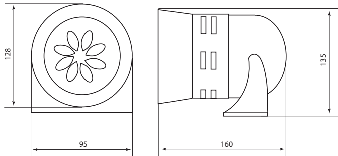
Рис. 1 - Сирена серии CC-1C
