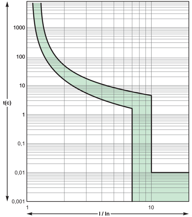
Кривая С
