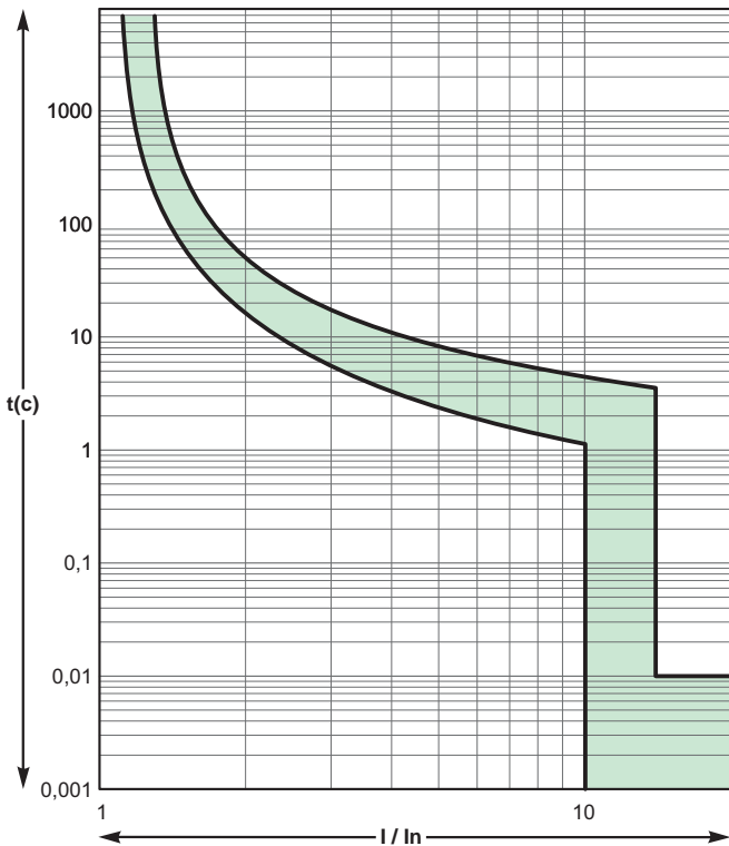
Кривая D
