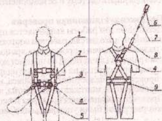
Рис. 1 1 - наплечная лячка 2 - пряжка ремня 3 - ремень 4 - D-кольцо (элемент крепления) 5 - набедр. лямки 6 - карабин 7 - фал стропа 8 - амортизатор 9 - кушак
